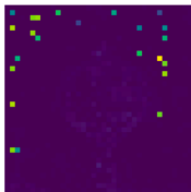
DINOv2-G
